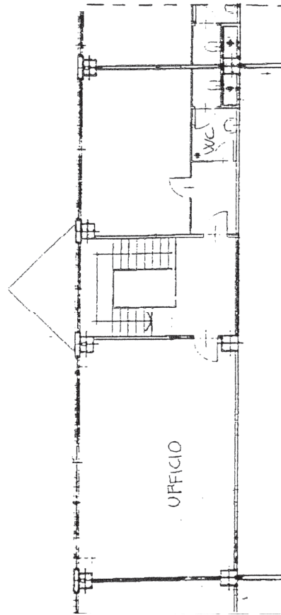
PIANO PRIMO
